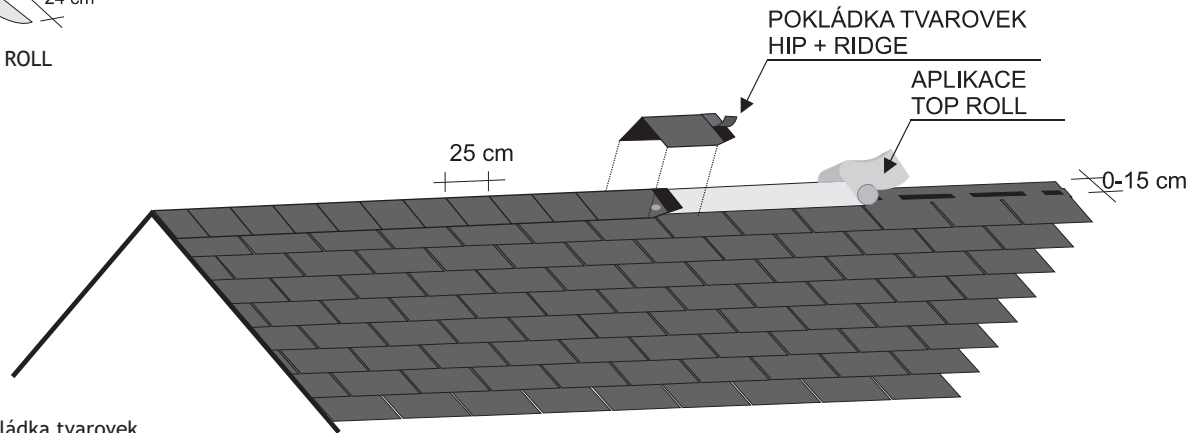
Obr. 9 - Pokládka tvarovek
