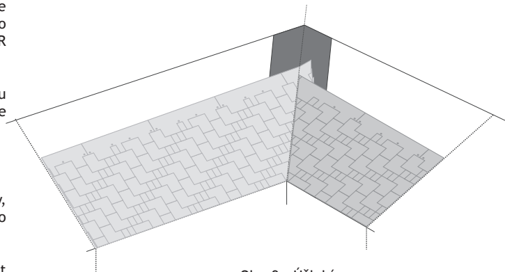
Obr. 9 - Úžlabí
