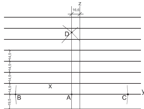
Obr. 1 - Rozvržení krytiny
