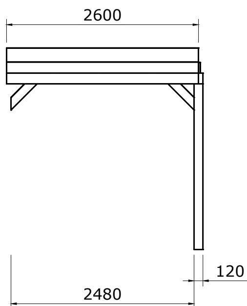
Vooraanzicht
