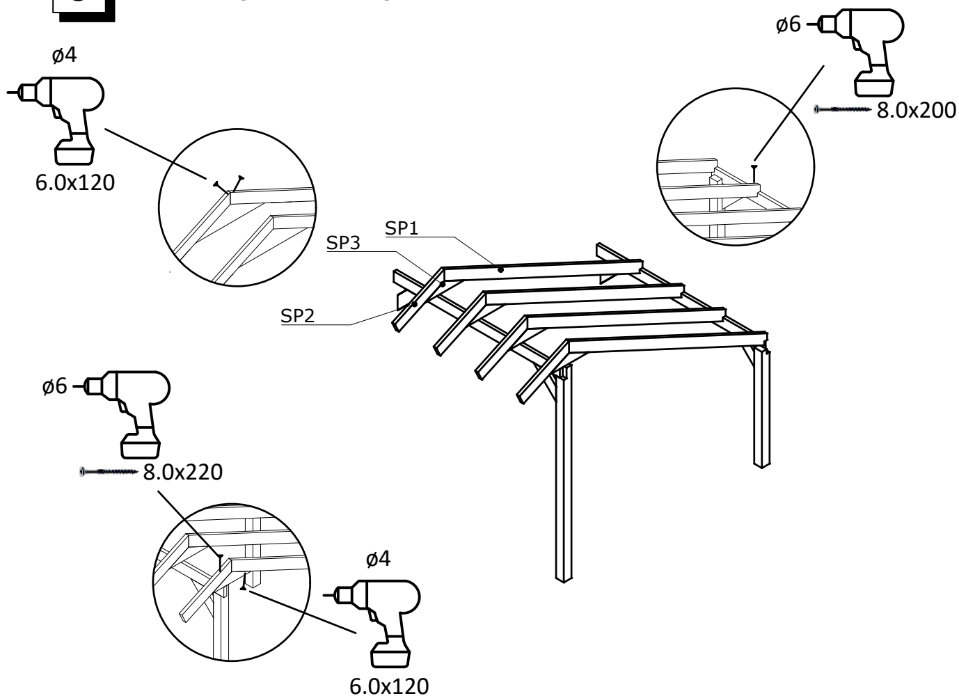
Bovenaanzicht
