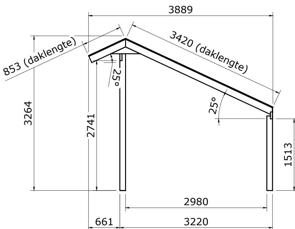
Rechter zijaanzicht
