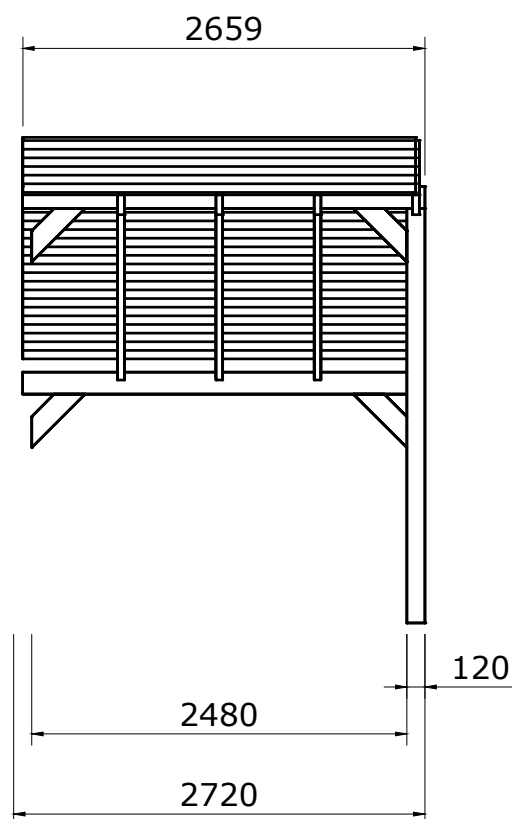
Vooraanzicht
