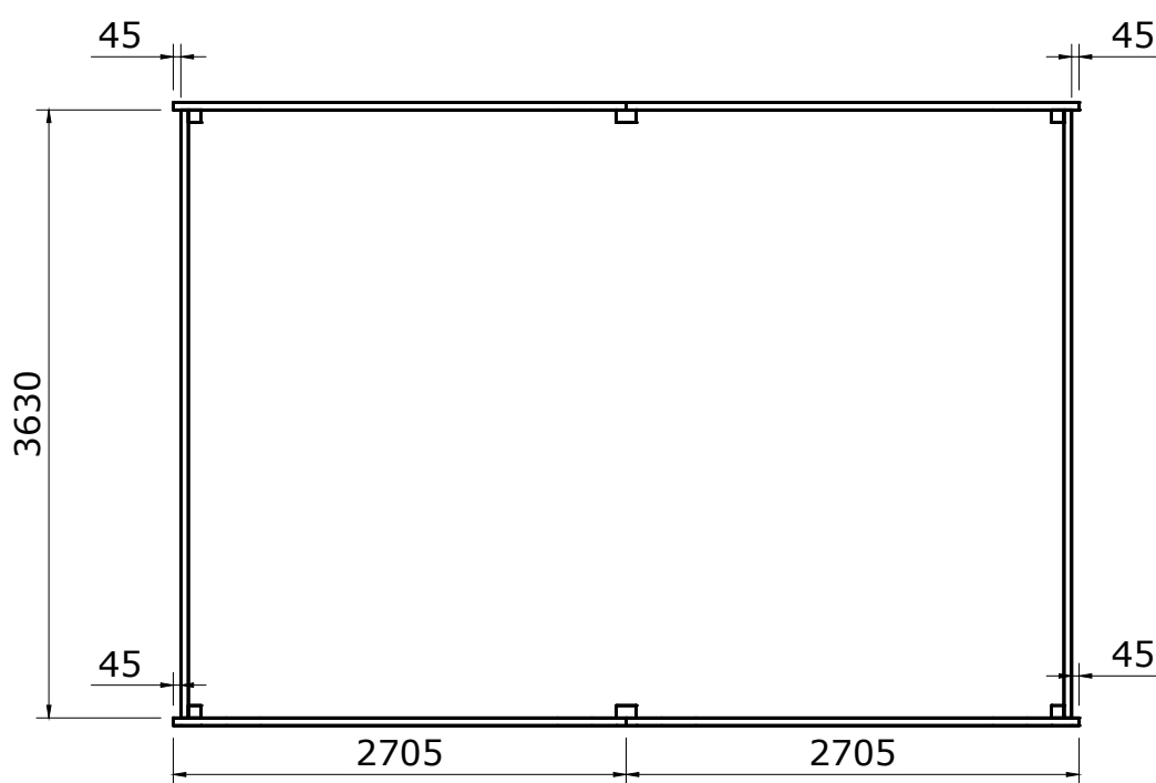
Bovenaanzicht
