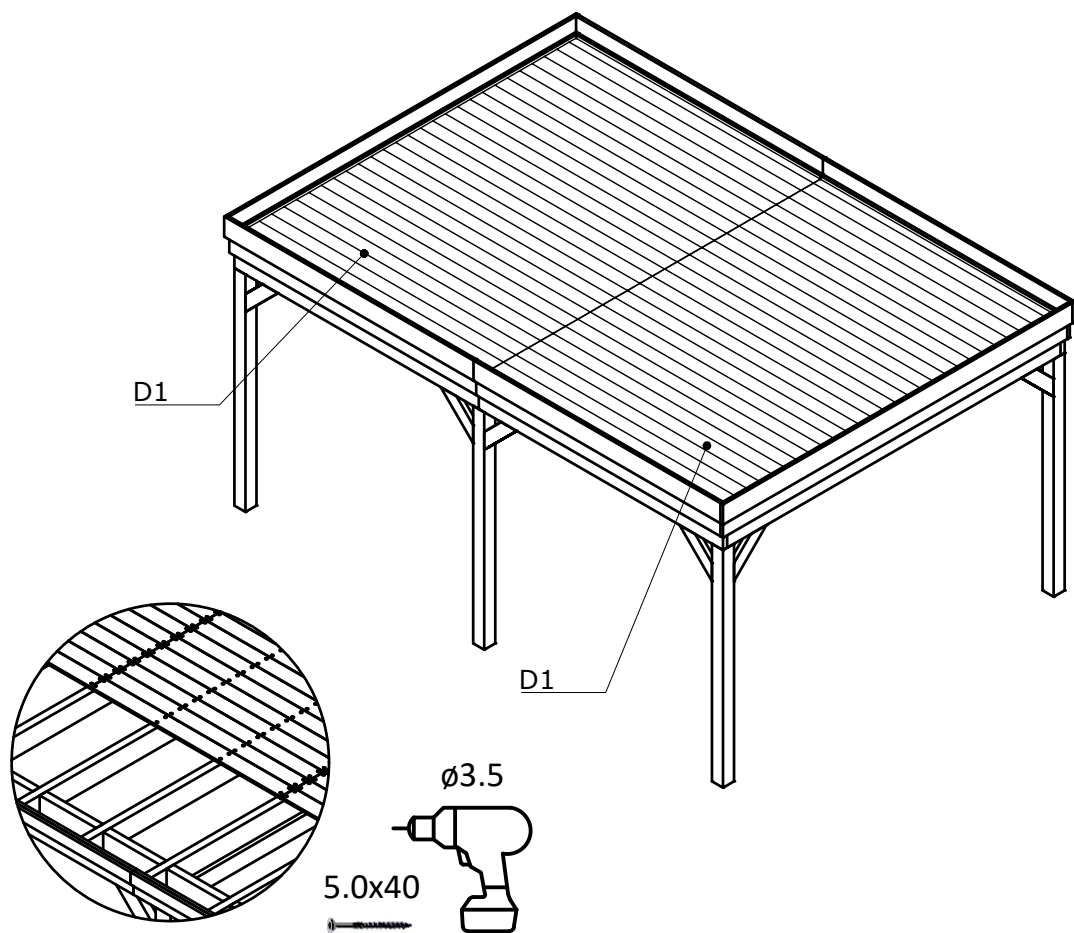
Bovenaanzicht
