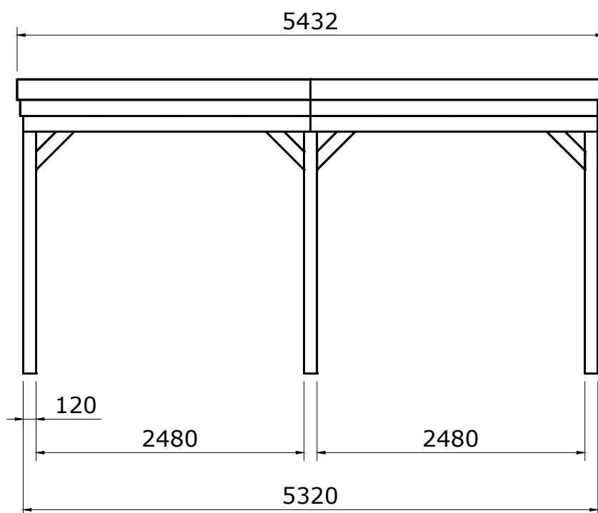
Vooraanzicht
